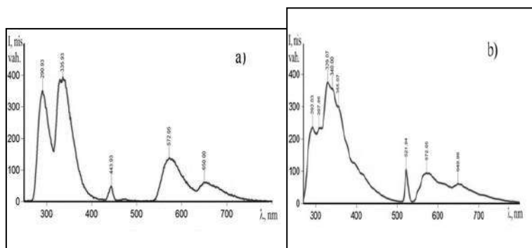
Şəkil 1. I AQK a) \lambda_{\text{həy.max.}} = 220 nm, b) \lambda_{\text{həy.max.}} = 266 nm lüminessent həyəcanlanma maksimumlarında lüminessensiya spektrləri
