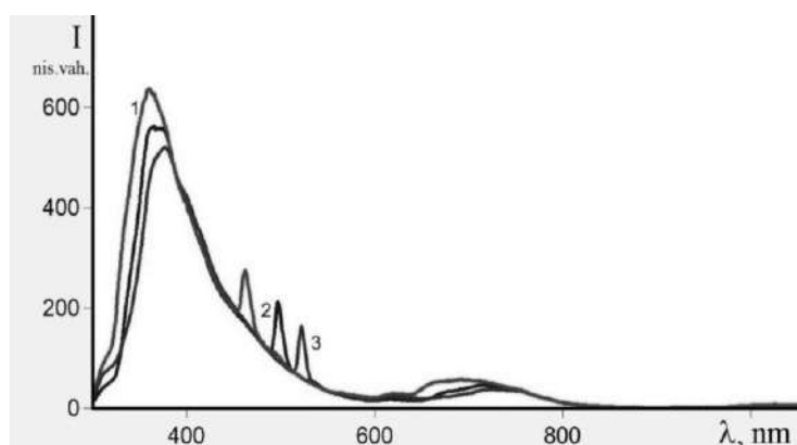
Şəkil 3. Ağır Suraxanı xam neftinin IV AQK komponentinin lüminessensiya spektrləri: 1\text{-}\lambda_{\text{həy.mak.}}=232 \text{ nm} , 2\text{-}\lambda_{\text{həy.mak.}}=250 \text{ nm} , 3\text{-}\lambda_{\text{həy.mak.}}=262 \text{ nm}
